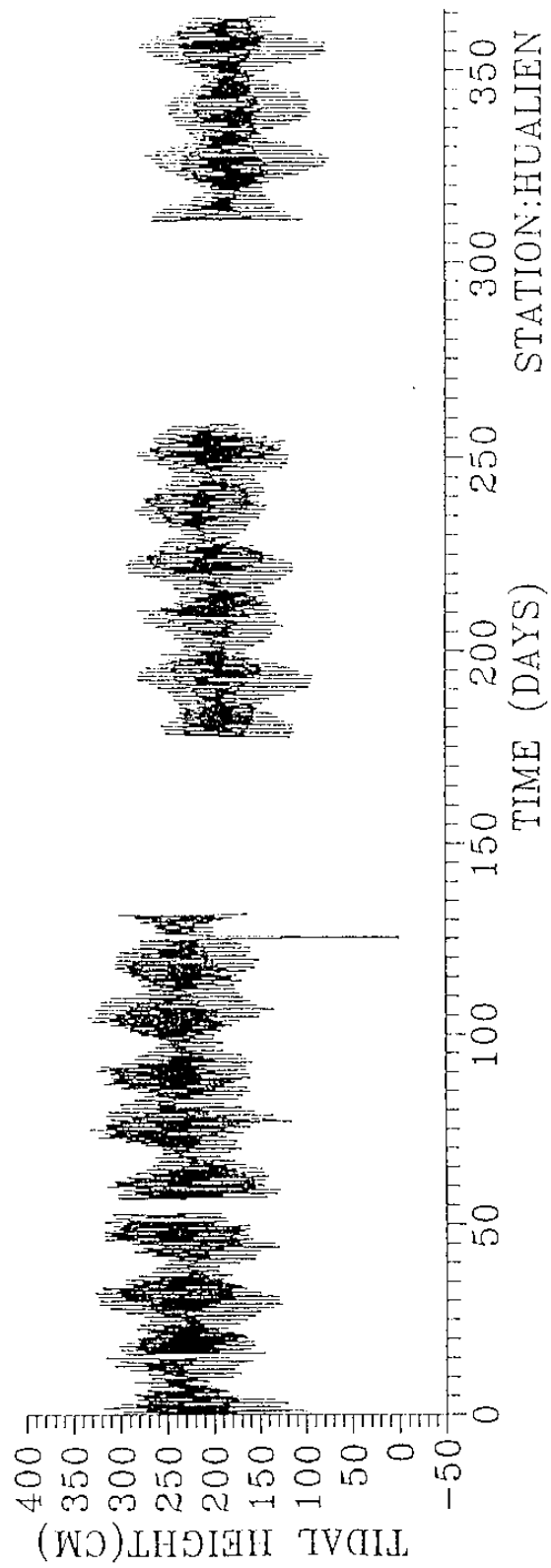
圖 2 f、蘇澳與花蓮之潮位圖。
