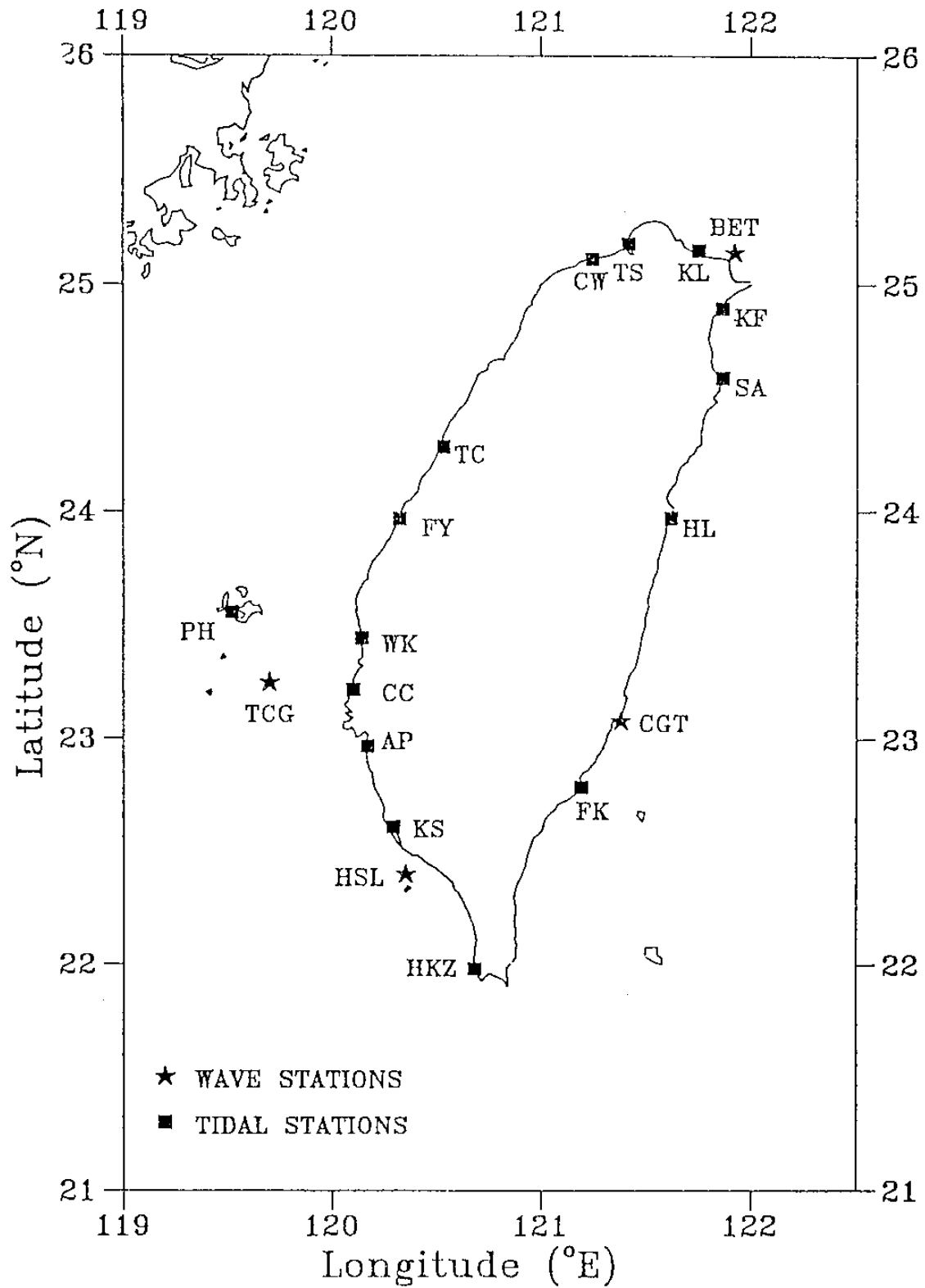
圖 1、全省之波浪站與潮位站。
